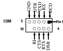
COM Header
